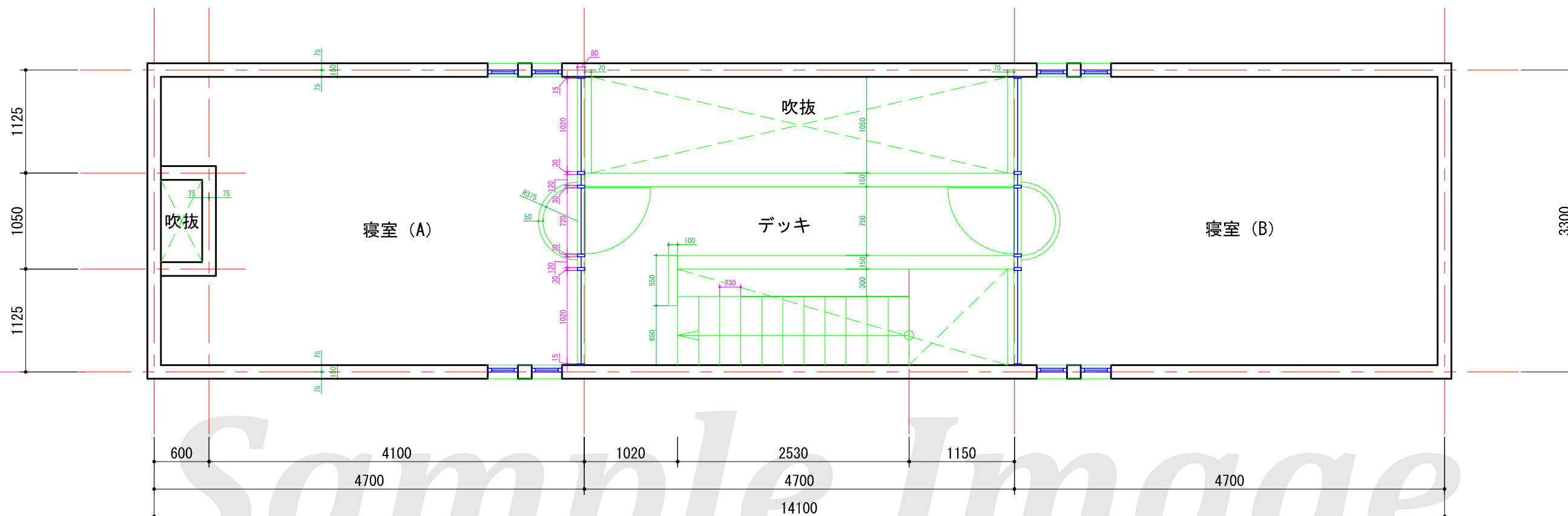
2階平面図
