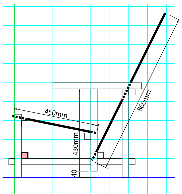
右面図
